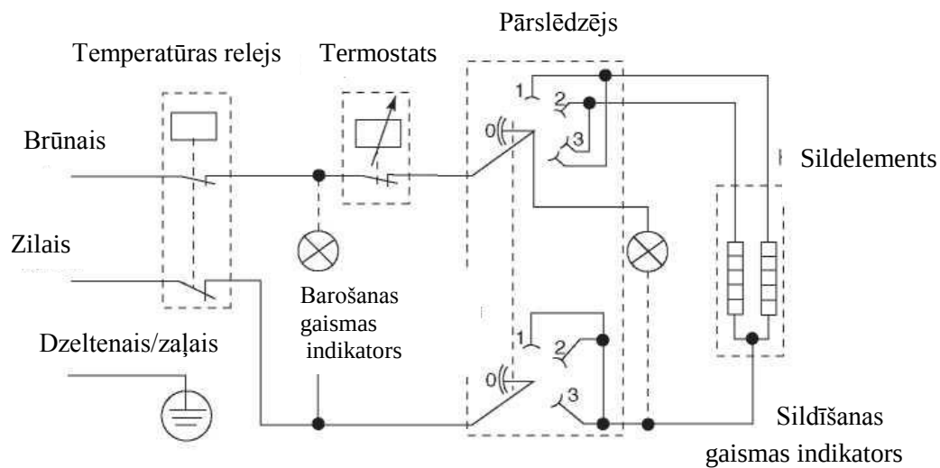
EWH Formax elektrosavienojumu shēma
